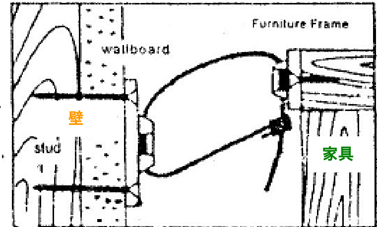
③壁側のブラケットと家具側のブラケットをバンドで留める。
